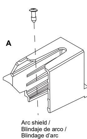
Figure / Figura / Figure 1 : Arc Shield and Arc Suppressor Housing / Blindaje de arco y caja de supresor de arco / Blindage d'arc et boîtier suppresseur d'arc
