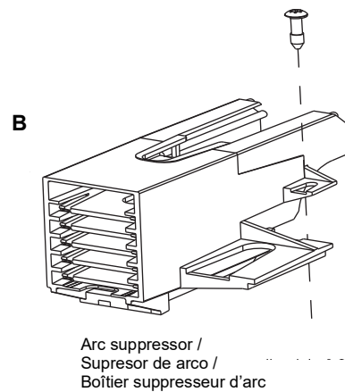
Figure / Figura / Figure 1 : Arc Shield and Arc Suppressor Housing / Blindaje de arco y caja de supresor de arco / Blindage d'arc et boîtier suppresseur d'arc
