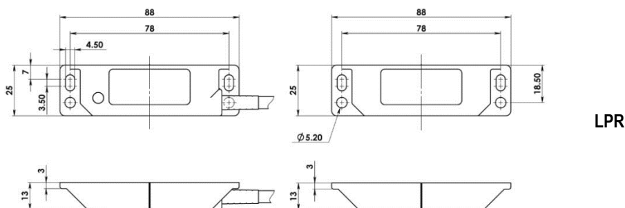
ACTUATOR
