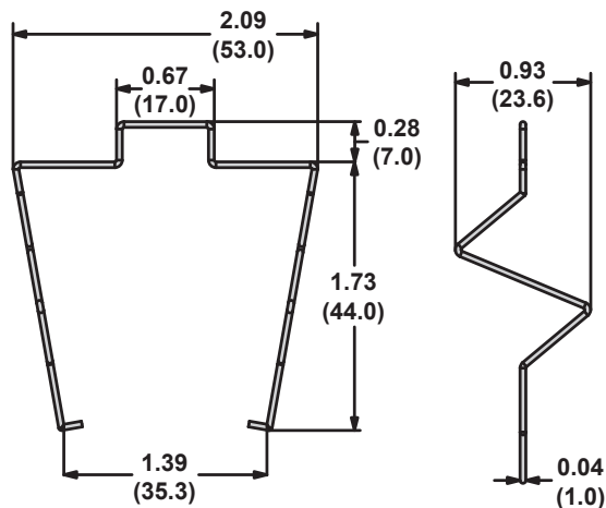
16-725SC
