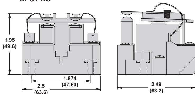
DPST-NO
