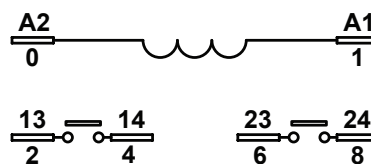
DPST-NO
