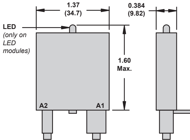
70-ASM Socket Modules
