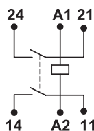
DPST-NO
